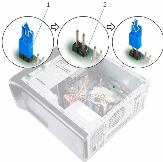
1 跳线塞
