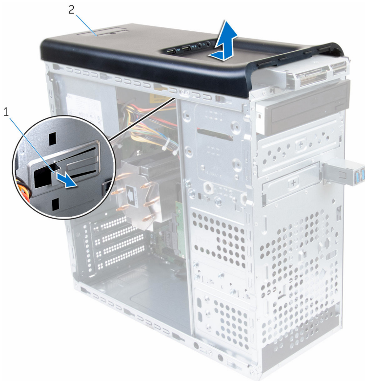
1 固定夹
